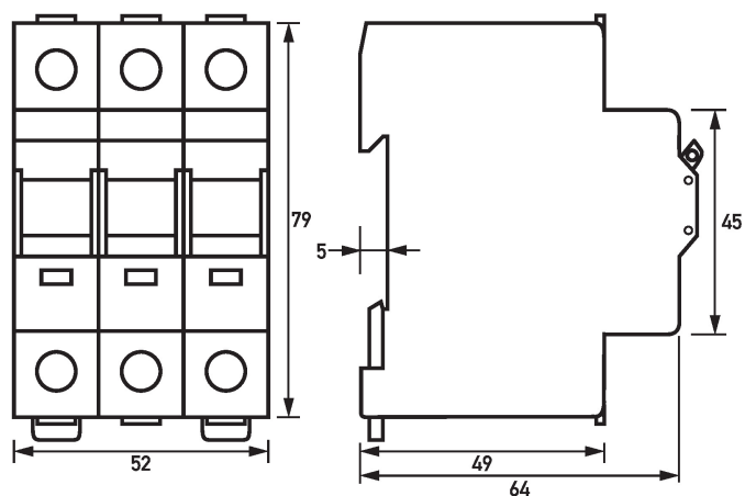
Rozměrový výkres RH (Celkový pohled)
